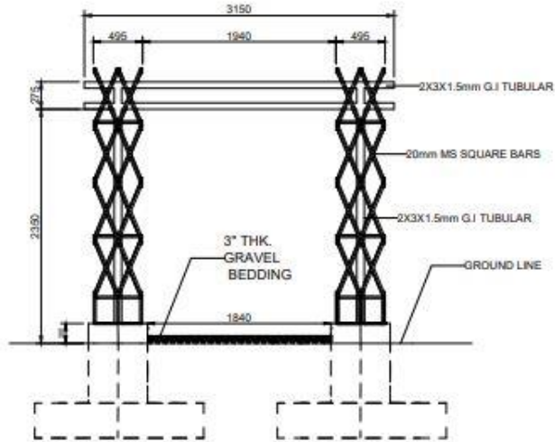
4 FRONT ELEVATION SCALE: 1:40M
