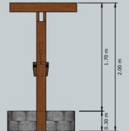
6 A5 SIDE ELEVATION scale: 1:20 M
