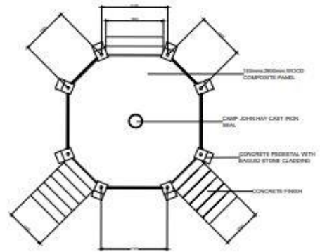
2 FLOOR PLAN SCALE: 1:100M
