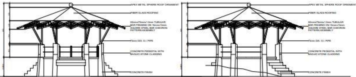
5 RIGHT SIDE ELEVATION SCALE: 1:100M
