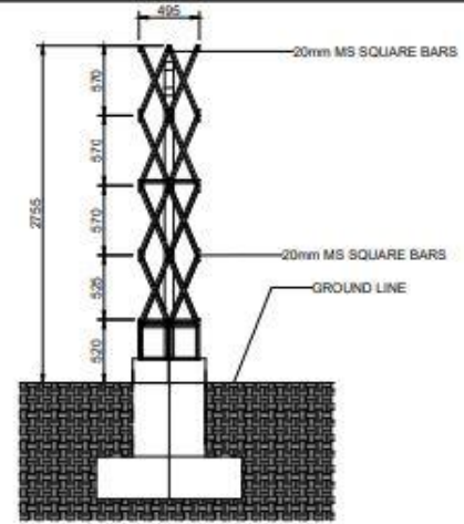
3 SIDE ELEVATION SCALE: 1:40M
