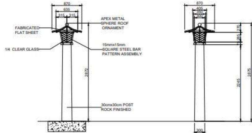
6 LAMP POST ELEVATION 1 SCALE: A10 1:40M
